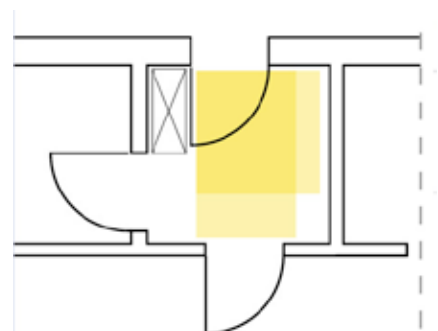
Bewegungsfläche bei Wohnungseingangstüren 1,40 m x 1,70 m oder 1,50 m x 1,50 m.
